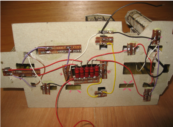
20 – Verdrahtung mit Pertinax-Leiterbahnplatten
